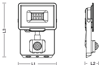
IS743-5-4000K
